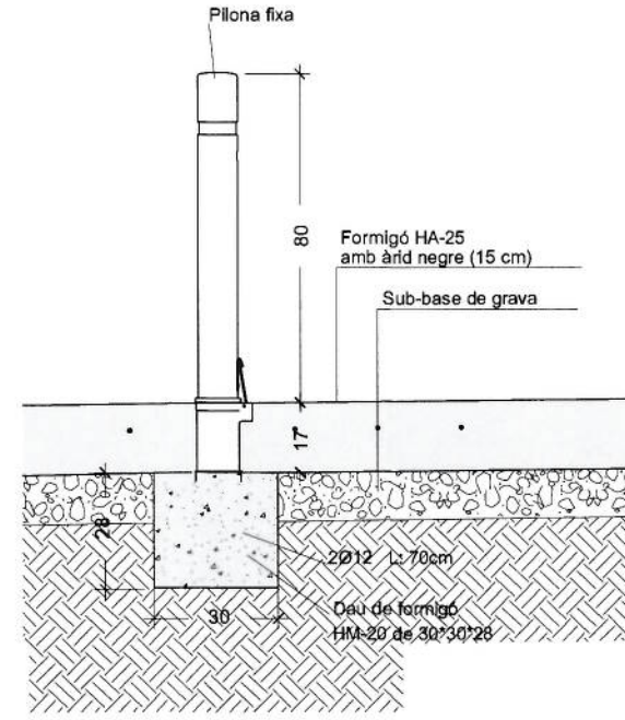
DETALLS OBRA CIVIL COL·LOCACIO PILONA EXTRAIBLE A1 e:1/10 A3 e:1/20
