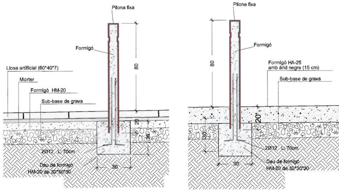
DETALLS OBRA CIVIL COL·LOCACIO PILONA FIXA A1 e:1/10 A3 e:1/20
