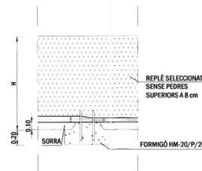
SECCIÓ C-C
