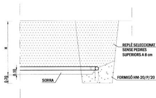
SECCIÓ A-A
