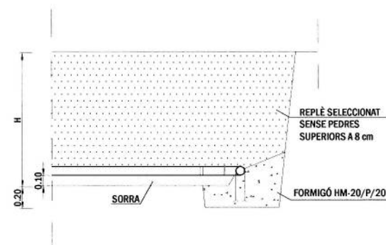
SECCIÓ B-B
