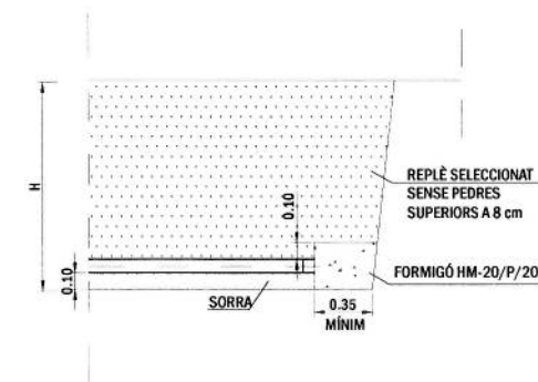
SECCIÓ D-D
