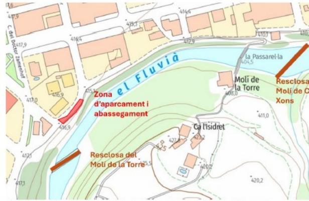
Figura 2. Zones d'estacionament de vehicles i acopi de materials relacionats amb el desenvolupament de l'obra
